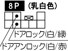
運転席ドアからきている ハーネスの中継カプラ
