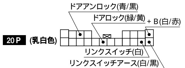
パワーウィンドウスイッチユニット
