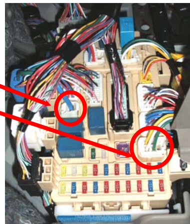
運転席足元のヒューズボックス部
