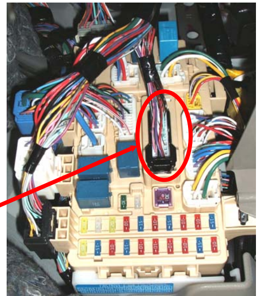
運転席足元のヒューズボックス部
