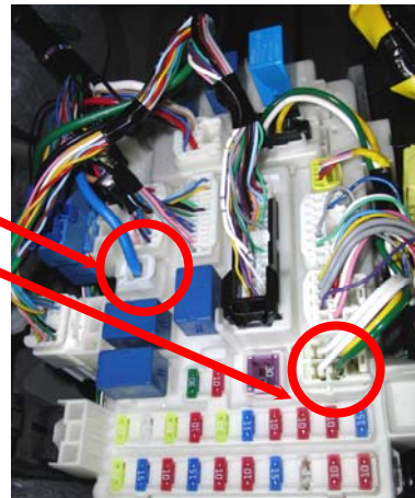
運転席足元のヒューズボックス部
