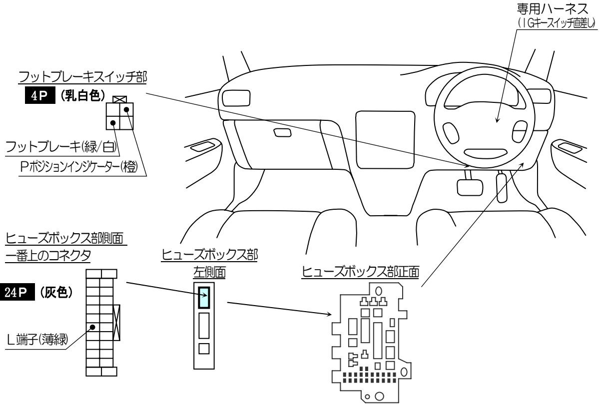
ヒューズボックス部正面
