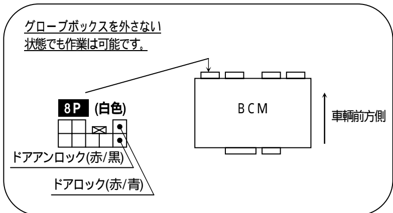
助手席グローボックス下 BCMユニットへ
