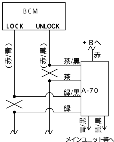
ドアロック接続
