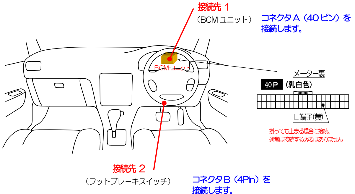
メーター裏にあるBCMユニット
